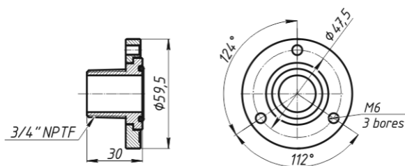
Adapter FP-ERL3/4-AA.
